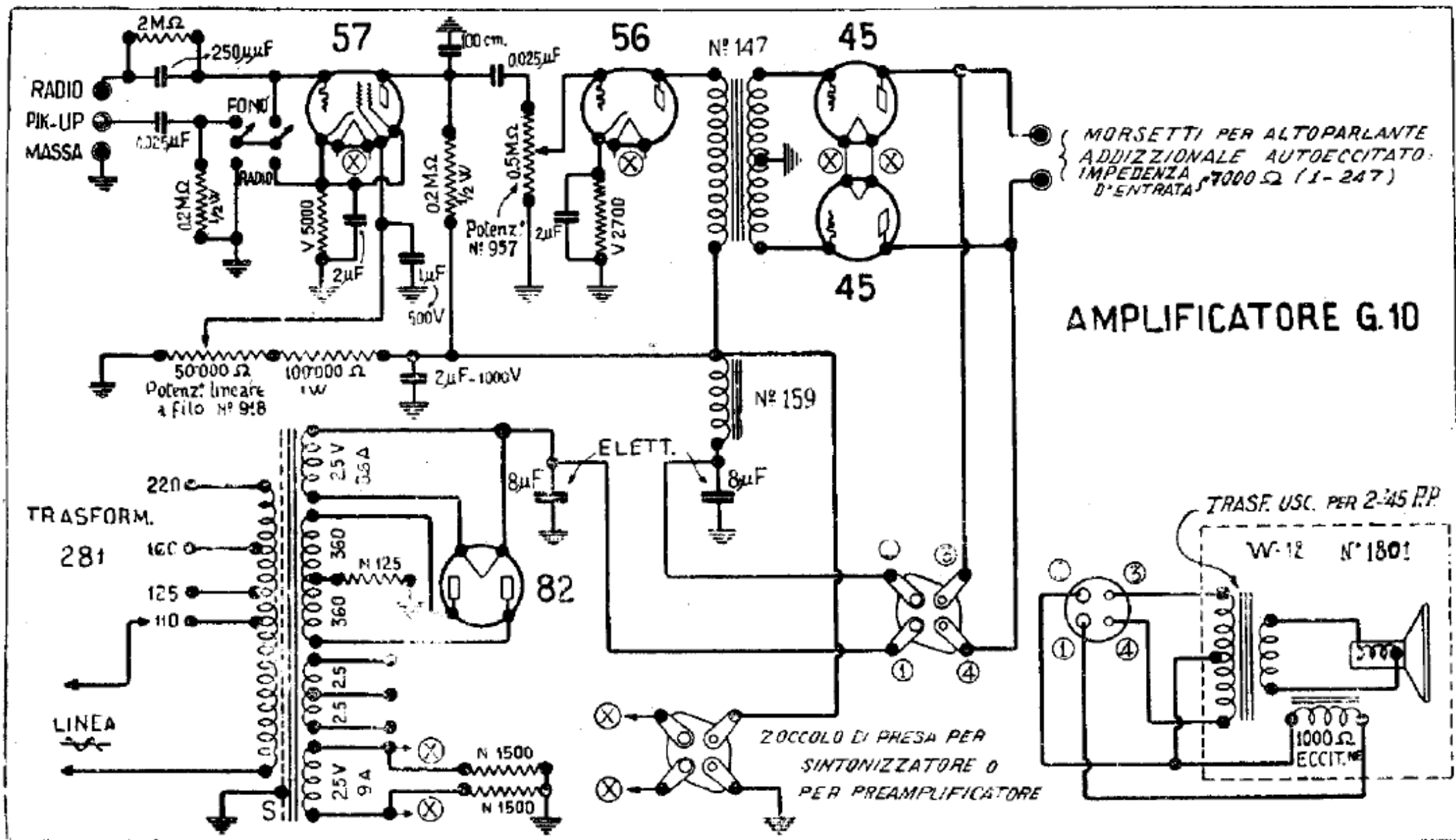
Schema elettrico dell'amplificatore G-10.
